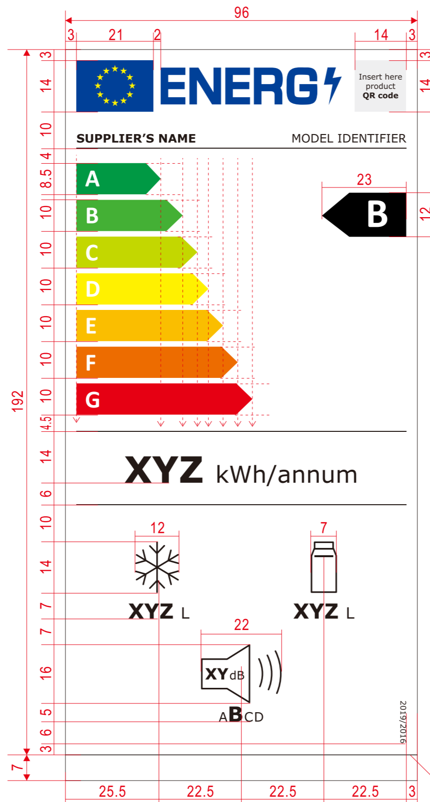
尺寸定位示意图
